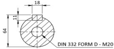
KESİT A-A
