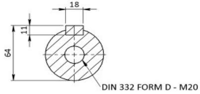
KESİT A-A
